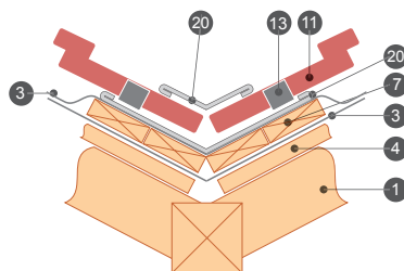
Устройство ендовы на стыках скатов
