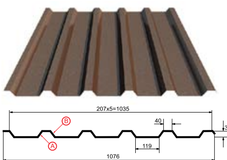
Профилированный лист МП-35x1035-В Толщина металла 0.5 - 0.9 мм
