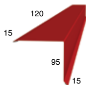
Планка торцевая 95x120x2000
