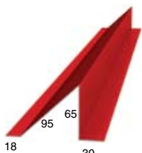
Планка снегодержателя 95x65x2000
