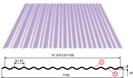
Профилированный лист МП-18x1100-А "Волна" Толщина металла 0.4 - 0.7 мм
