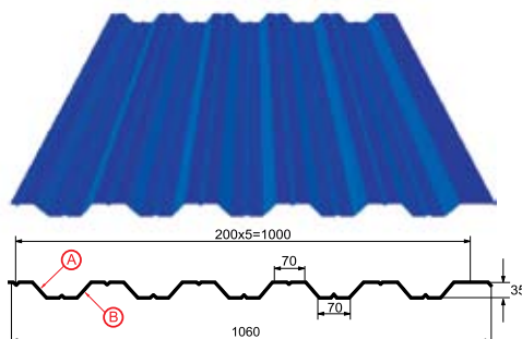
Профилированный лист НС-35x1000-А Толщина металла 0.5 - 0.9 мм
