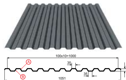
Профилированный лист С-21x1000-А Толщина металла 0.4 - 0.7 мм
