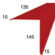
Планка торцевая 135x145x2000
