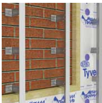
Крепежные кронштейны КК-50 (90, 120, 150, 180 и 230), с шайбой и изоляционной прокладкой, t=1.2 и 2.0 мм
