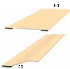
Планка стыковочная 60x3000 Планка начальная сайдинга 10x20x3000 (для сайдинга "Корабельная доска")
