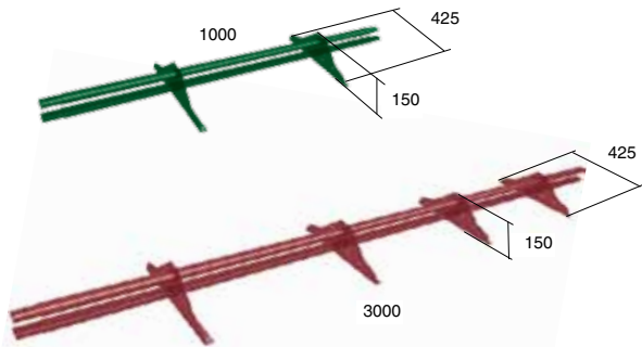
Снегозадержатели трубчатые СЗТ-h150x3000, СЗТ-h150x1000
