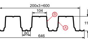
Профилированный лист Н-114х600-А,В Толщина металла 0.8 - 1.0 мм
