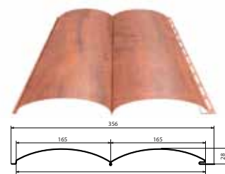
Стальной сайдинг Woodstock-28x330
