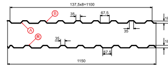
Профилированный лист МП-20х1100-А,В,Р Толщина металла 0.4 - 0.8 мм
