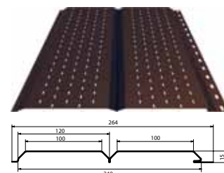
Софит Лбрус (перфорированный) для подшивки карнизных свесов
