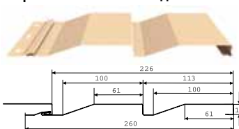
Стальной сайдинг МП СК-14x226
