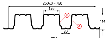
Профилированный лист Н-114х750-А,В Толщина металла 0.8 - 1.0 мм
