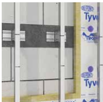
Крепежные кронштейны межэтажные ККМ-90 (120, 150, 180 и 230), t=1.2 и 2.0 мм
