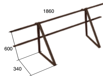
Ограждение кровельное ОК- h600x1860
